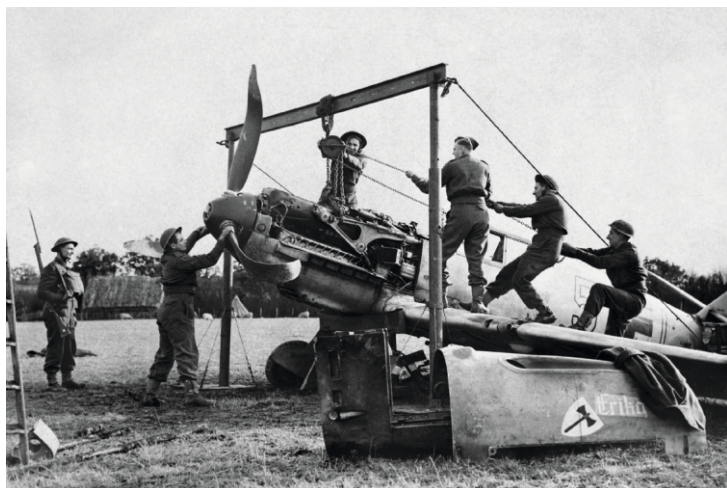
Staffelkapitán 9./JG 3 Oblt. Egon Troha byl s tímto Bf 109E-4 zajat 29. října 1940 po boji se Spitfirů 74. squadrony. Letoun původně patřil Lt. Franzu Achleitnerovi, jenž padl do zajetí s jiným strojem 24. srpna. Foto: IWM via Wikimedia Commons
